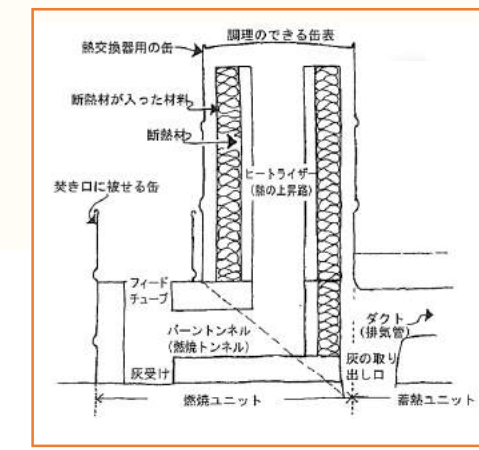
ロケットストーブの中はこうなっています
